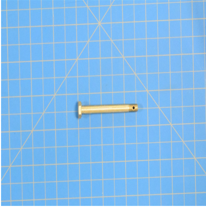
NAS6604D32 - Bolt
